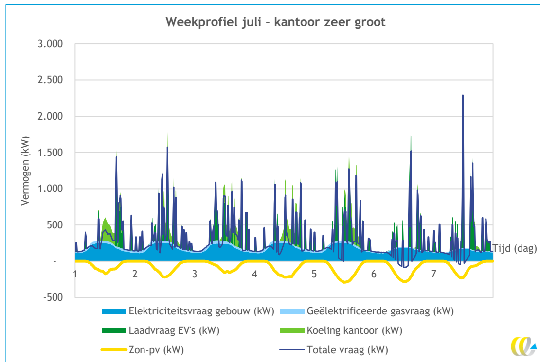
Figuur 30 - Elektricitetsvraag van de casus zeer groot kantoor voor de eerste week van juli
