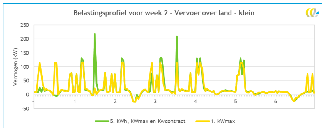
Figuur 16 - Effect van tariefvariant 1 en 5 in voorbeeldwijk - vervoer op land klein
