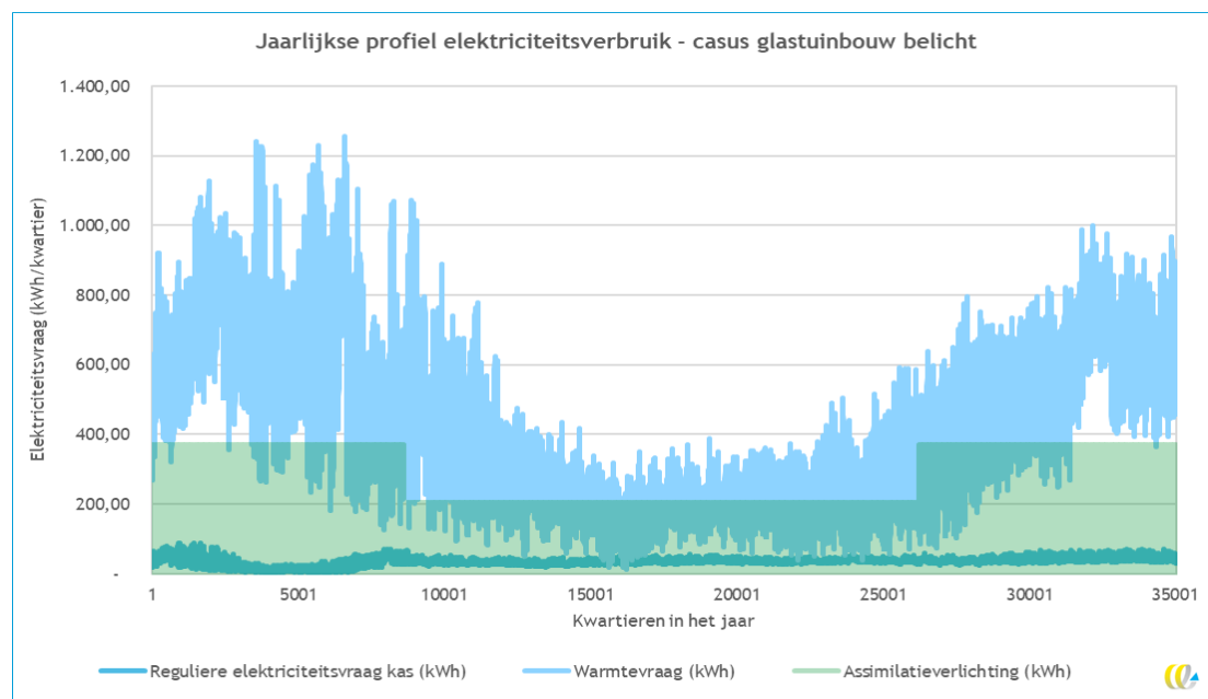
Figuur 99 - Elektriciteitsvraag van glastuinbouw in een heel jaar. De geëlektrificeerde gasvraag is 70% van de gasvraag zonder elektrificatie van de warmtevoorziening. De overige 30% van de originele gasvraag wordt met de wkk omgezet in warmte, elektriciteit en CO 2 ..
