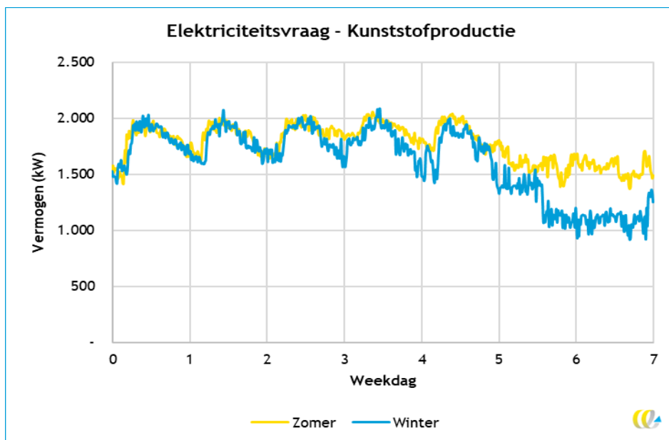
Figuur 159 - Weekprofielen van de kunststoffenproductie.
