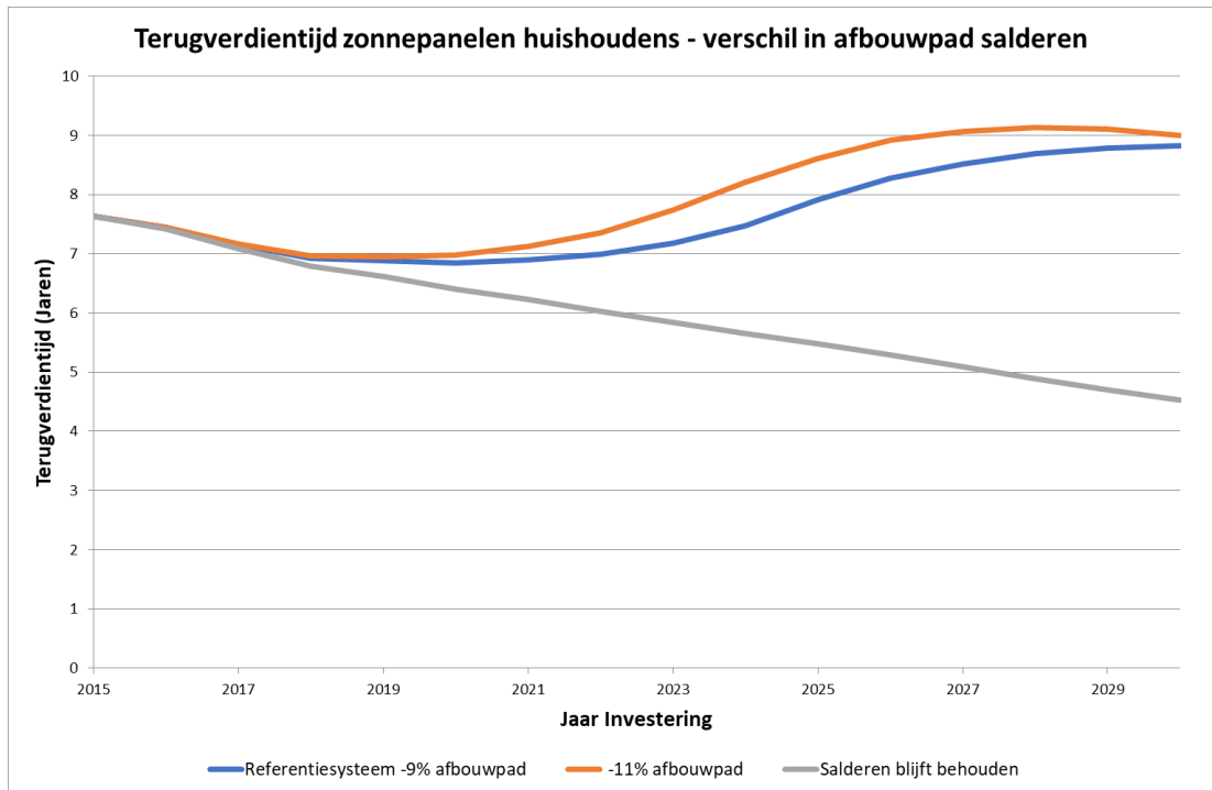
Figuur 2. Terugverdientijd voor het referentiesysteem bij verschillende afbouwpaden van salderen: -9% afbouwpad, -11% afbouwpad en een pad waarbij de huidige regeling ook vanaf 2023 blijft bestaan.
